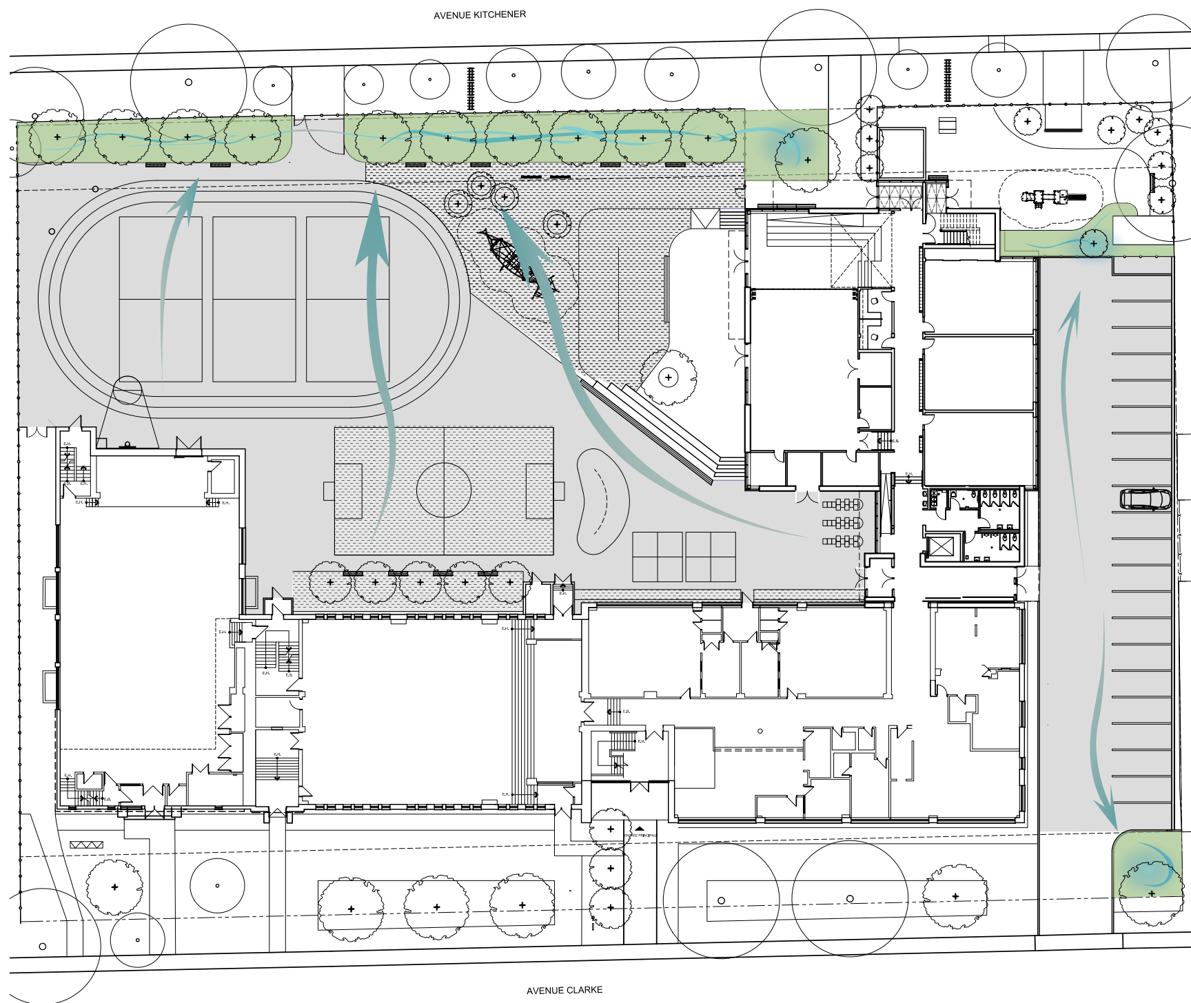
1. Diagramme de gestion des eaux pluviales
